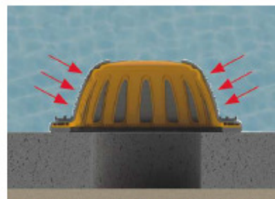
bacino pieno ; la falda si ritira e la valvola trattiene l'acqua
