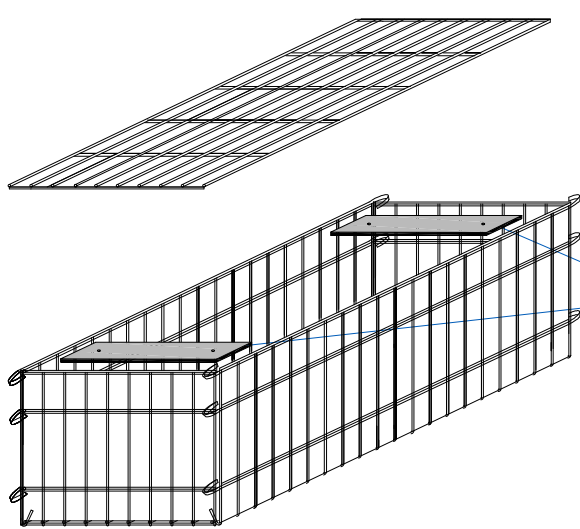
STEP 16 Coperchio
